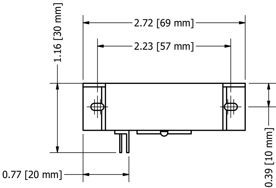
CTI-200 SCALE 1 : 1
